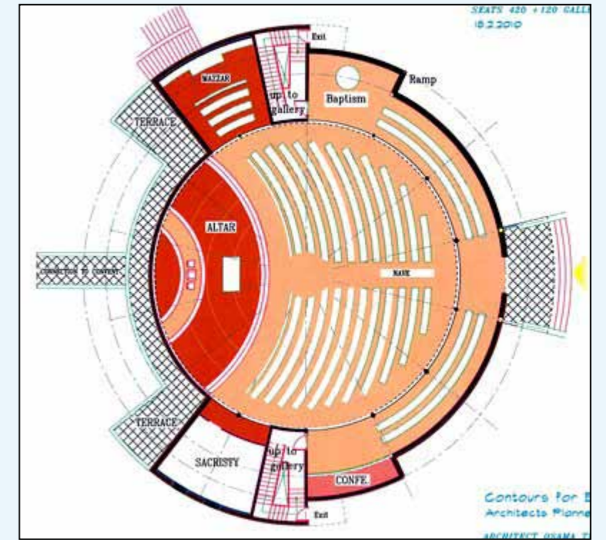
Plan intérieur du complexe paroissial Stella Maris
